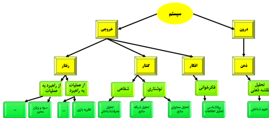
نمودار ۱. نمودار چگونگی بهره‌مندی از جدول درک نیت
