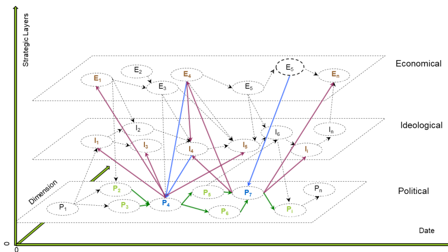
نمودار ۳. نمودار تحلیل اطلاعات محاسباتی در بستر فضای اقلیدسی
